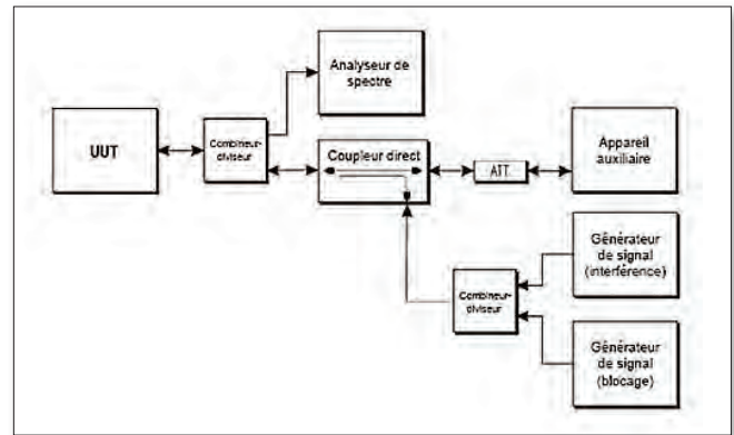
FIGURE 2 : Montage de test pour le test d'adaptabilité et de blocage du récepteur
