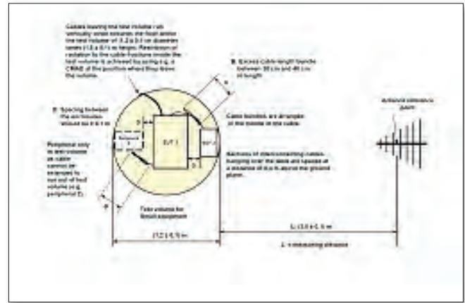
Rys.4. Stanowisko pomiarowe wraz z anteną z [4].
