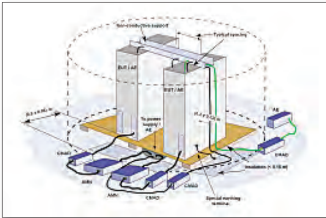
Rys.3. Stanowisko pomiarowe dla urządzeń podłogowych z [4].
